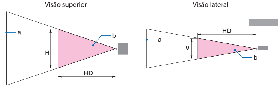
a: Tela / b: Zona de perigo
