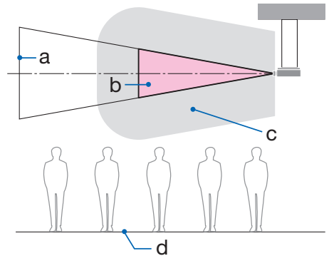
a: Tela / b: Zona de perigo / c: Zona de precaução / d: piso
