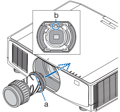
a: 돌출부 / b: 가이드 노치
