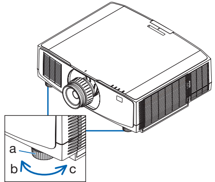
a: Lutningsfot / b: Upp / c: Ned
