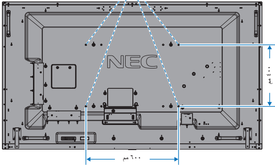
واجهة تثبيت متوافقة مع معايير (M8)
