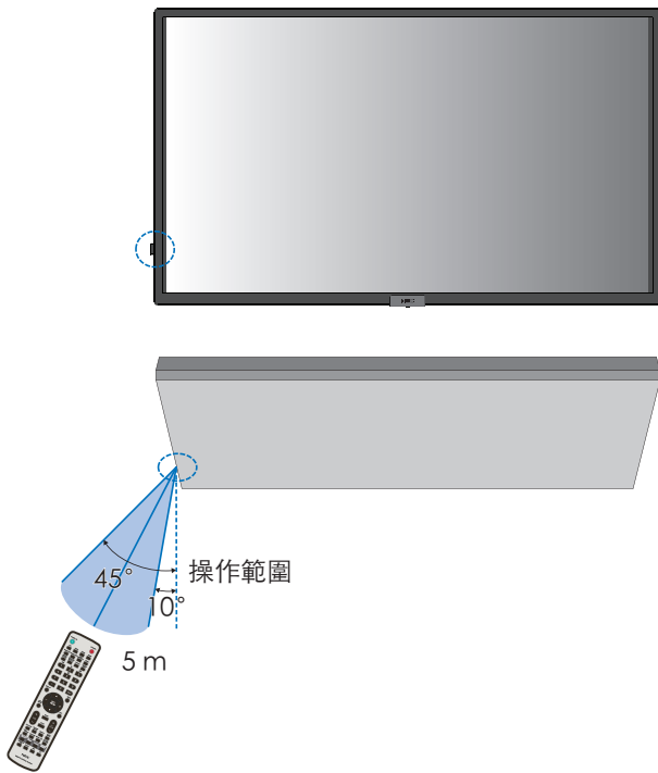
橫向時的操作範圍
