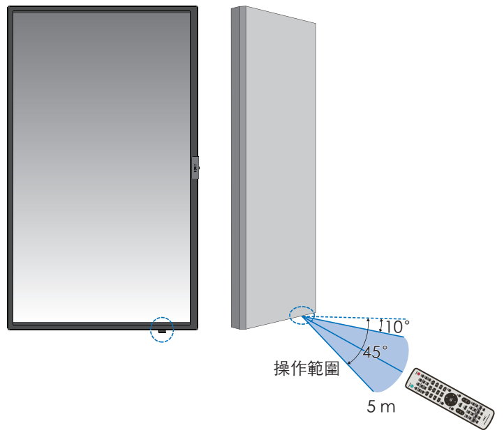
垂直方向時的操作範圍
