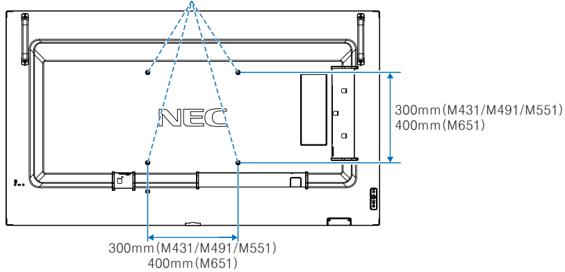
VESA 마운트 인터페이스 M6(M431/M491/M551), M8(M651)
